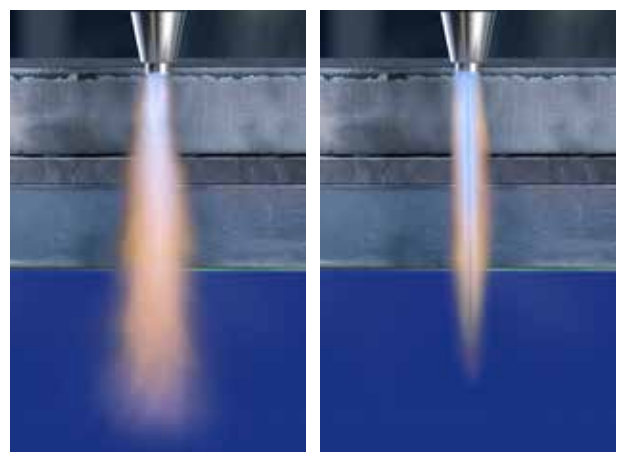
Frei brennende Wasserstoff-Sauerstoff-Flamme, optimal eingestellt (links) und Flamme mit zugeschaltetem Schneidsauerstoff (rechts)
